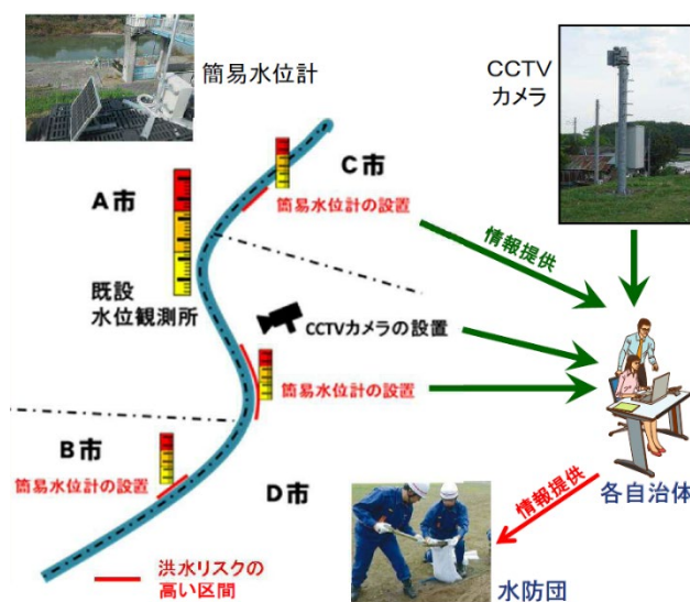
水害リスクが高い箇所でリアルタイムに水位を把握するための簡易水位計の設置
