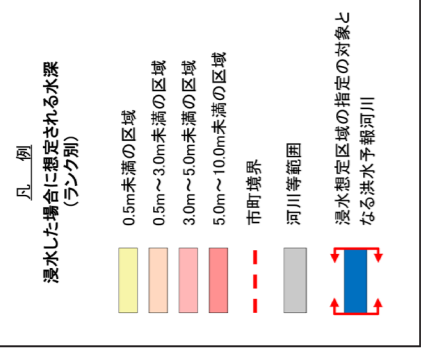
淀川水系淀川・宇治川・木津川・桂川洪水浸水想定区域図(1) (想定最大規模)
