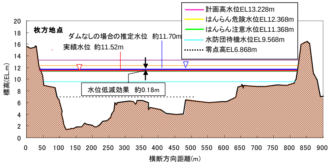
図 2.3-8 枚方地点水位低減効果
