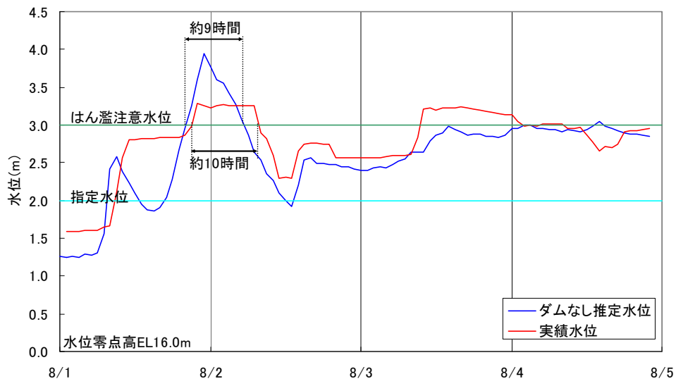
図 2.3-9 昭和 57 年(1982 年)8 月（台風 10 号）槇尾山地点労力低減効果
