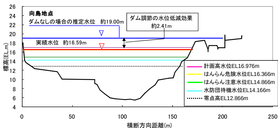
図 2.3-7 向島地点水位低減効果
