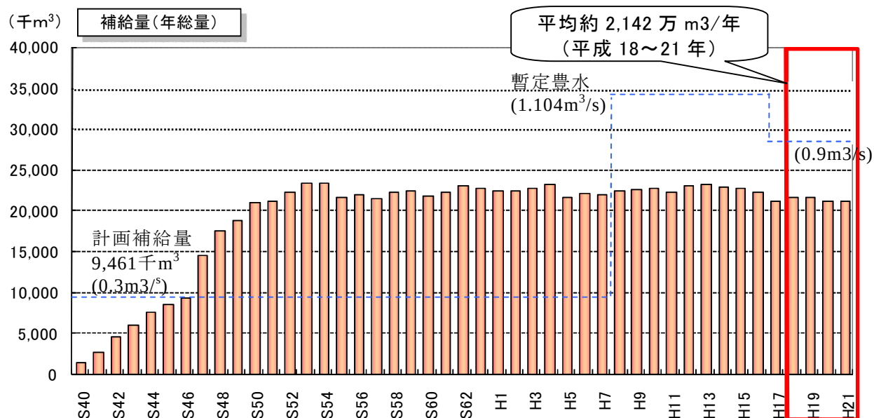
図 3.3-7 水道補給実績図
