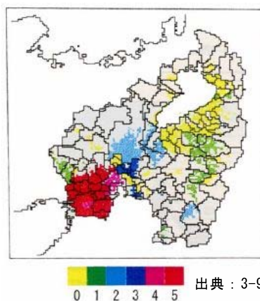
図 3.3-4 河川水の反復利用回数
