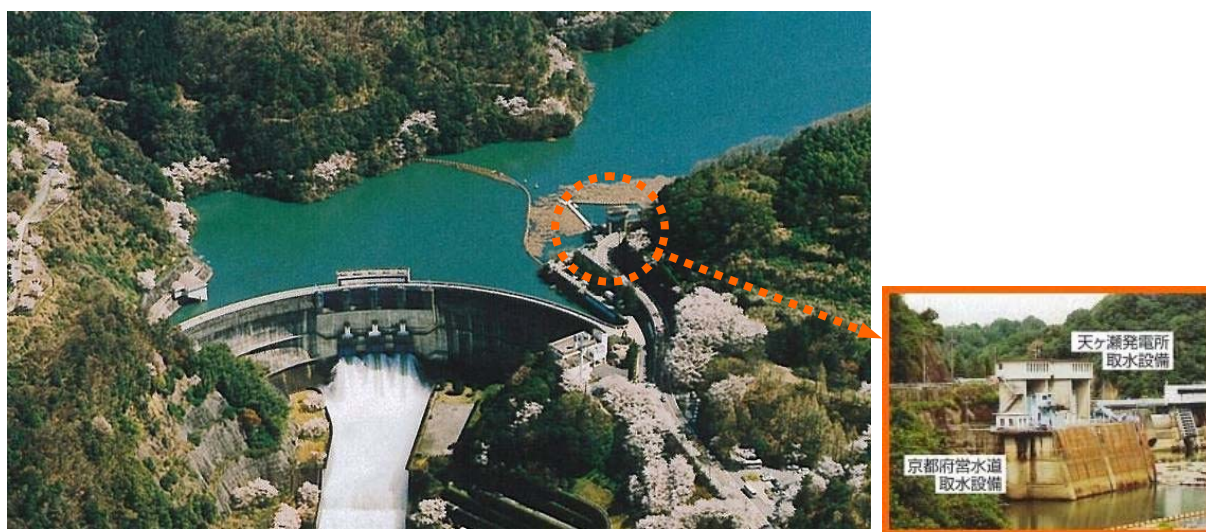
図 3.2-3 ダム地点取水設備
