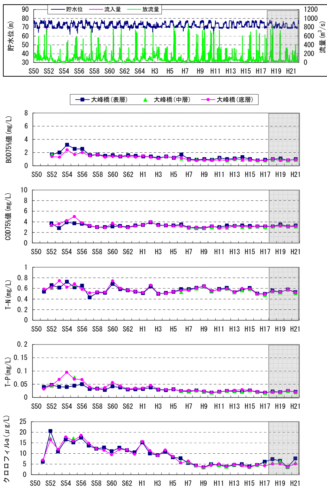
図 5.3-16(2) 貯水池水質の経年変化(大峰橋)
