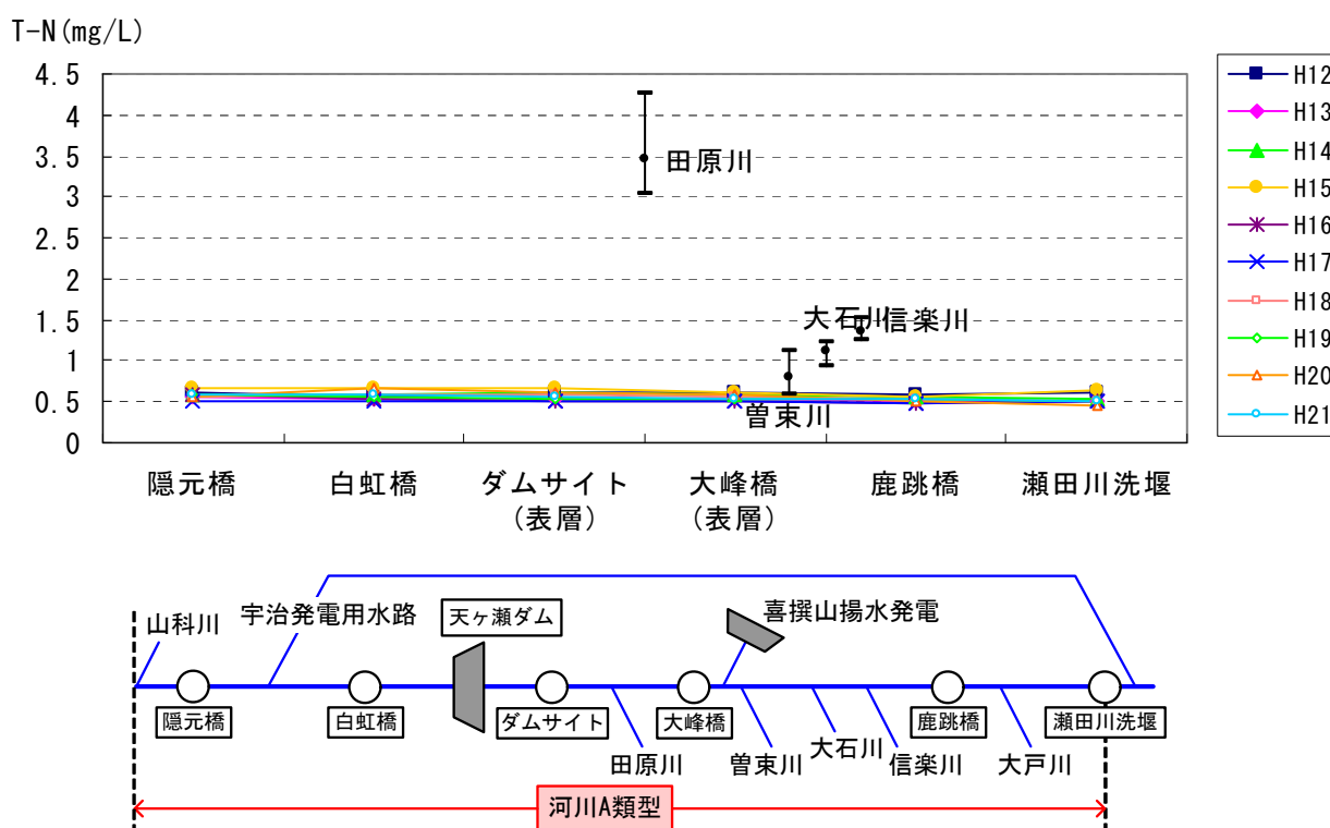
図 5.5-35 天ヶ瀬ダム年平均 T-N 濃度の縦断変化
