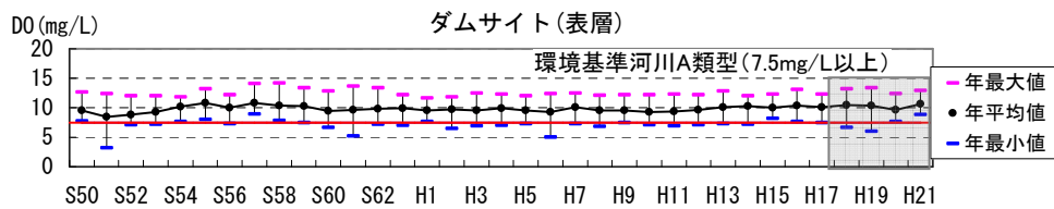
図 5.3-15(3) ダムサイト地点表層 DO 年平均値の経年変化
