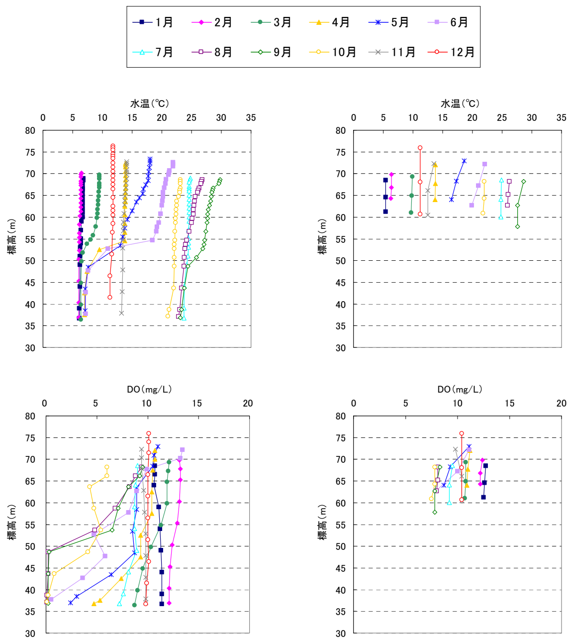
図 5.3-20(2) ダムサイト及び大峰橋地点 水温・DO の水質鉛直分布(平成 19 年)
