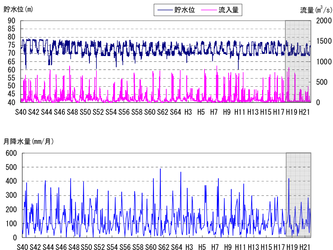
図 5.3-1 ダム諸量と天ヶ瀬ダム管理支所月降水量
