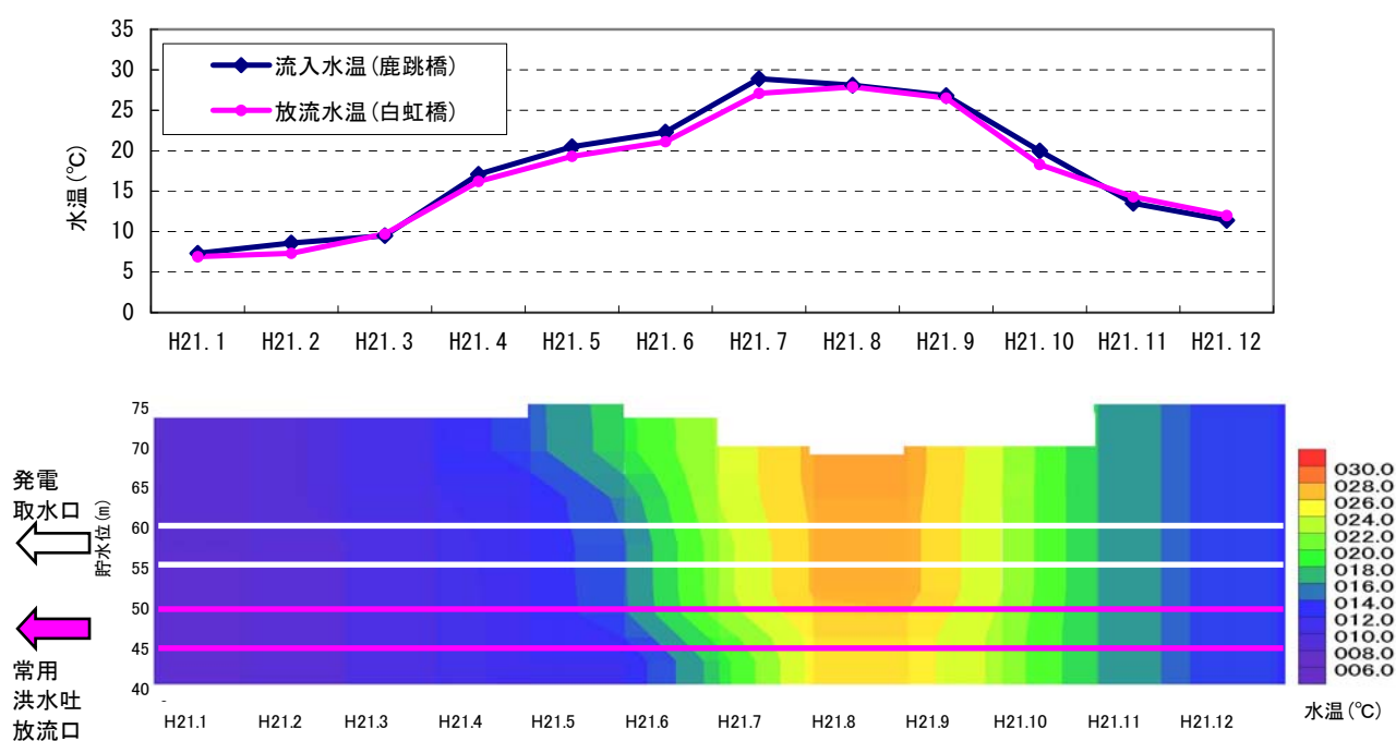
図 5.5-4 貯水池水温分布と流入・放流水温の比較(平成 21 年)
