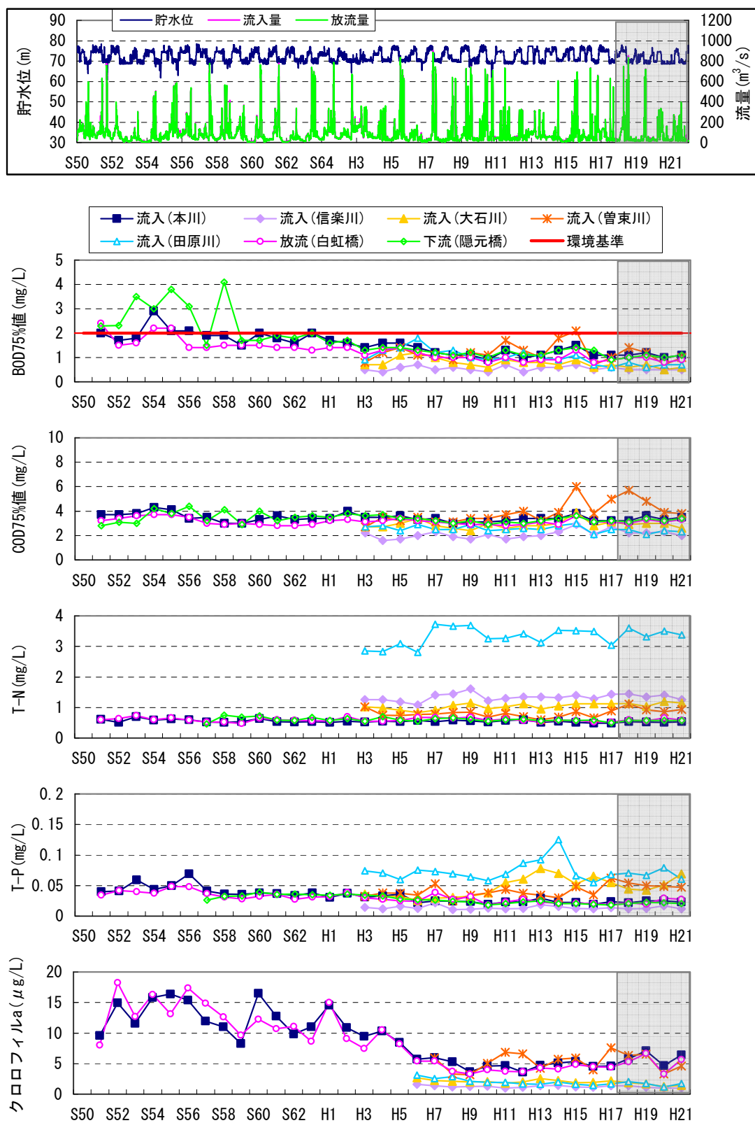
図 5.3-11(2) 流入・放流水質の経年変化
