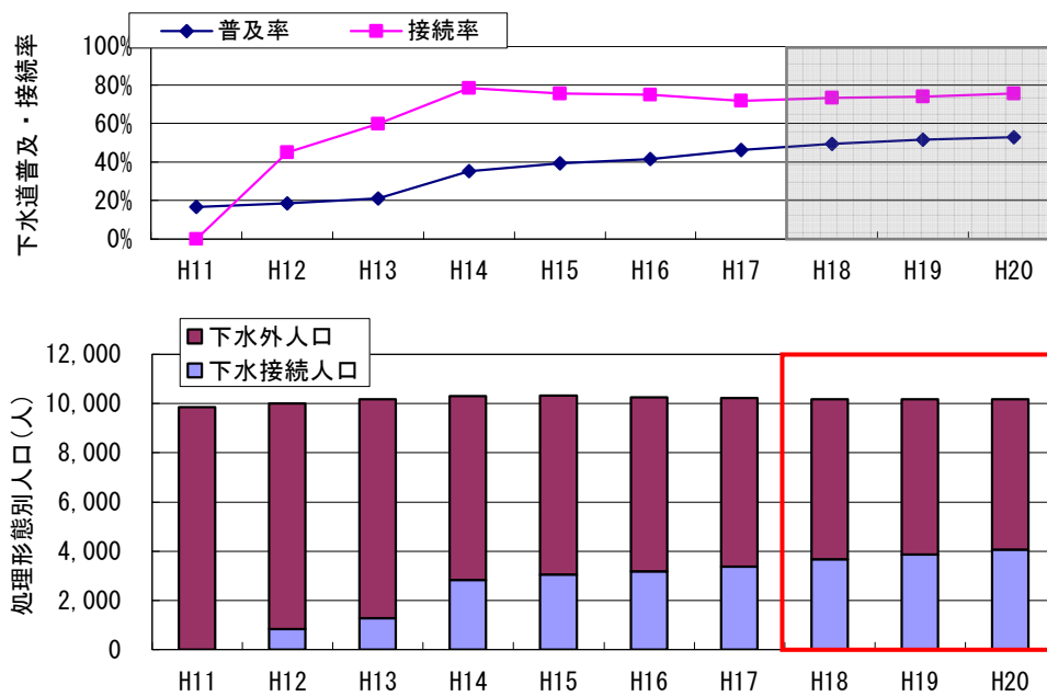
図 5.4-7 排水処理状況の変化(佐賀県域)
