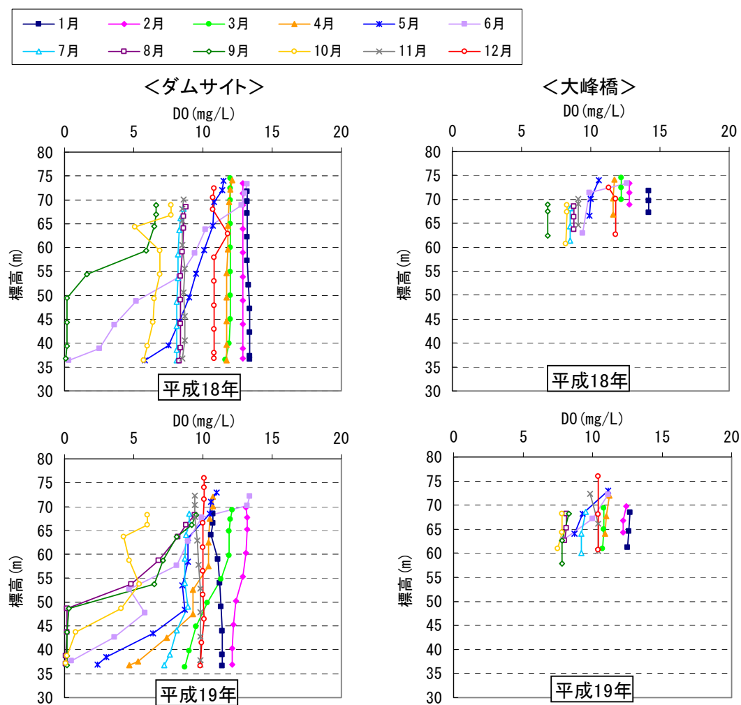
図 5.5-22(1) D0 鉛直分布図(平成 18 年～19 年)
