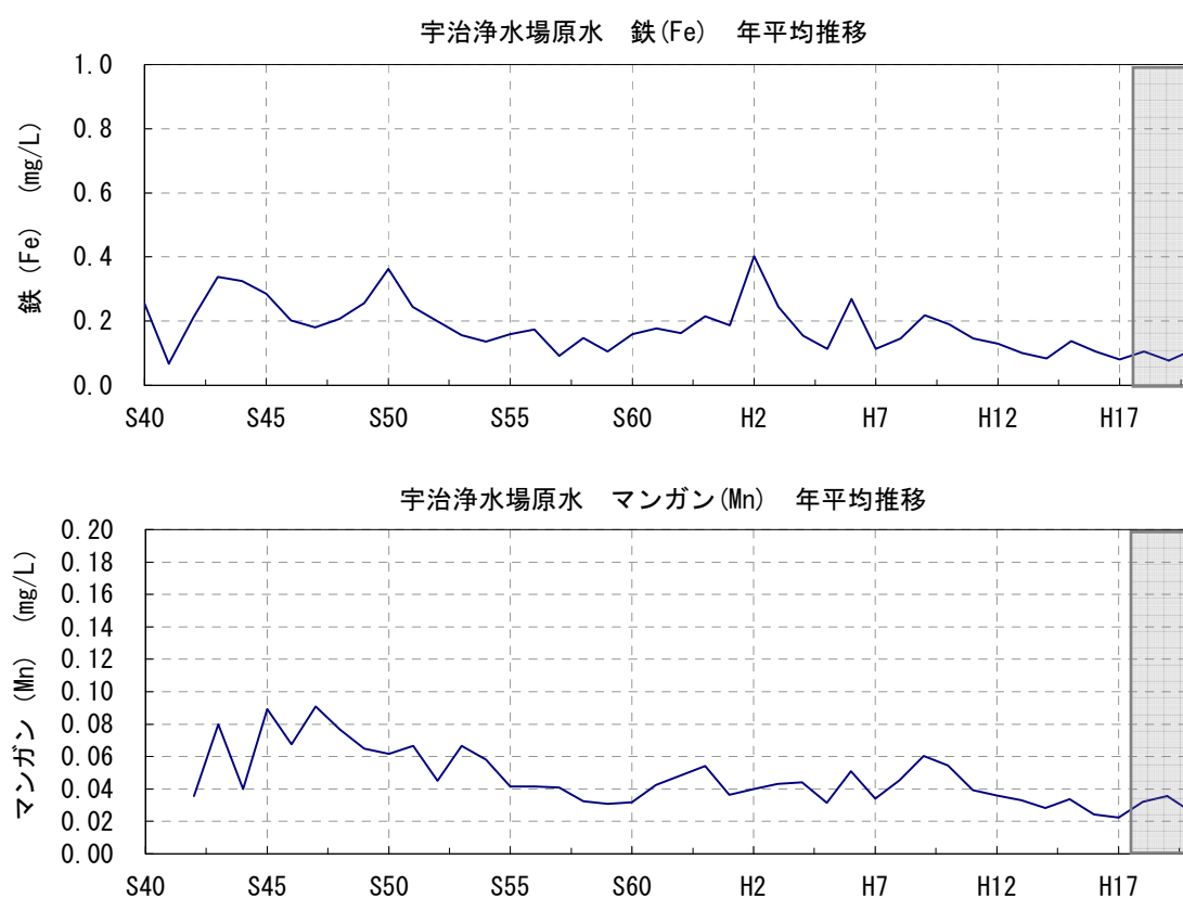
図 5.5-24 宇治浄水場原水の鉄・マンガン分析結果 出典：宇治浄水場提供データ
