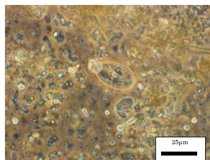
珪藻綱 Cocconeis placentula (コクコネイス プラセンツラ) 撮影条件：対物レンズ40倍 撮影レンズ5倍
