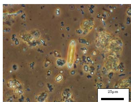
珪藻綱 Navicula cryptocephala (ナビキュラ クリプトセファラ) 撮影条件：対物レンズ40倍 撮影レンズ5倍
