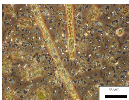
珪藻綱 Aulacoseira granulate (アウレコシラ グラヌラータ) 撮影条件：対物レンズ20倍 撮影レンズ5倍
