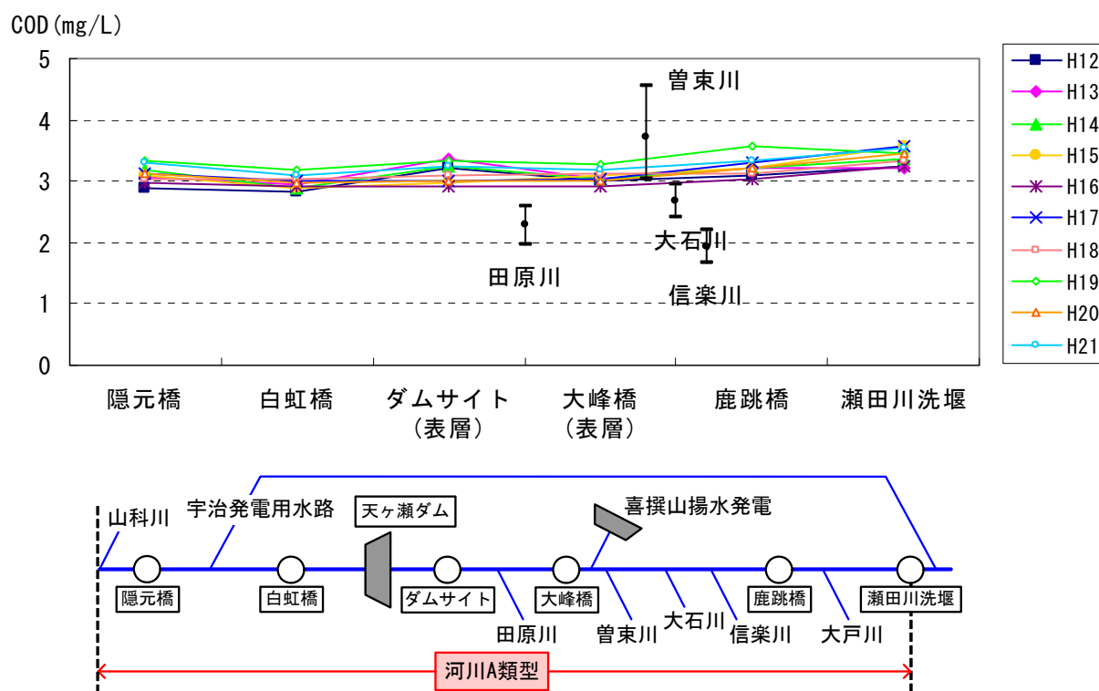
図 5.5-34 天ヶ瀬ダム COD 年平均値の縦断変化
