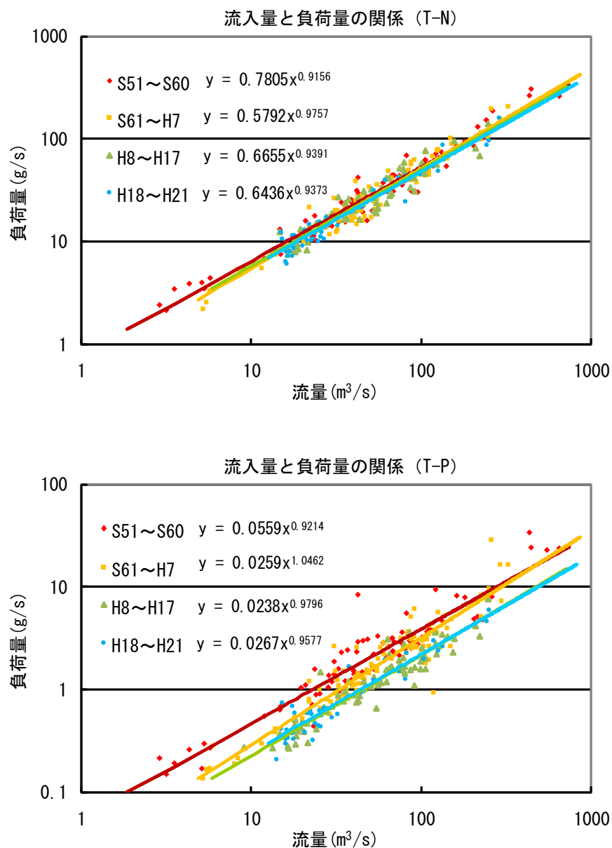
図 5. 3-36 (2) 流入本川の流入量と負荷量の関係 (T-N、T-P)
