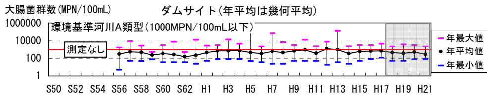
図 5.3-15(6) ダムサイト地点表層大腸菌群数年幾何平均値の経年変化 (幾何平均 G_m = (\prod X_i)^{1/n} で算定している)
