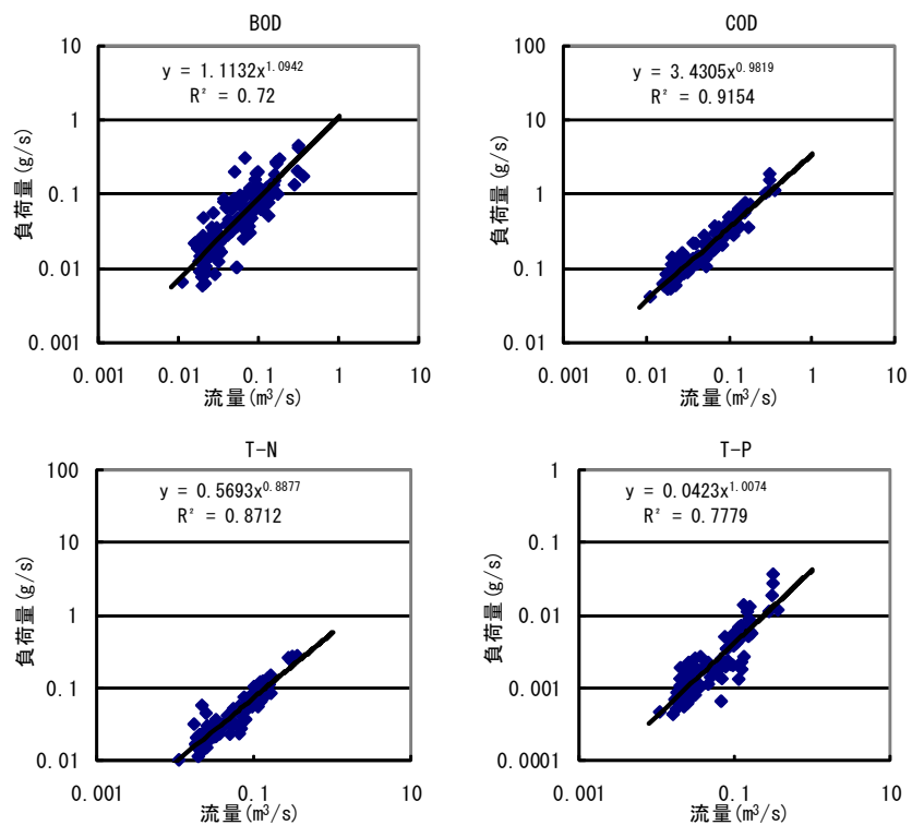
図 5.3-38 曾束川の流量と負荷量の関係
