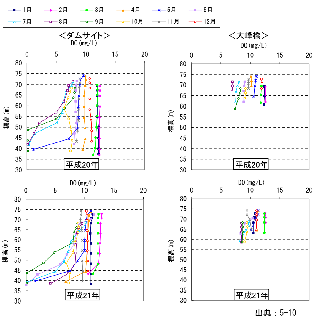
図 5.5-22 (2) DO 鉛直分布図 (平成 20 年～21 年)
