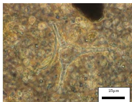
緑藻綱 Staurostrum 属(スタウラスツルム属) 撮影条件：対物レンズ40倍 撮影レンズ5倍
