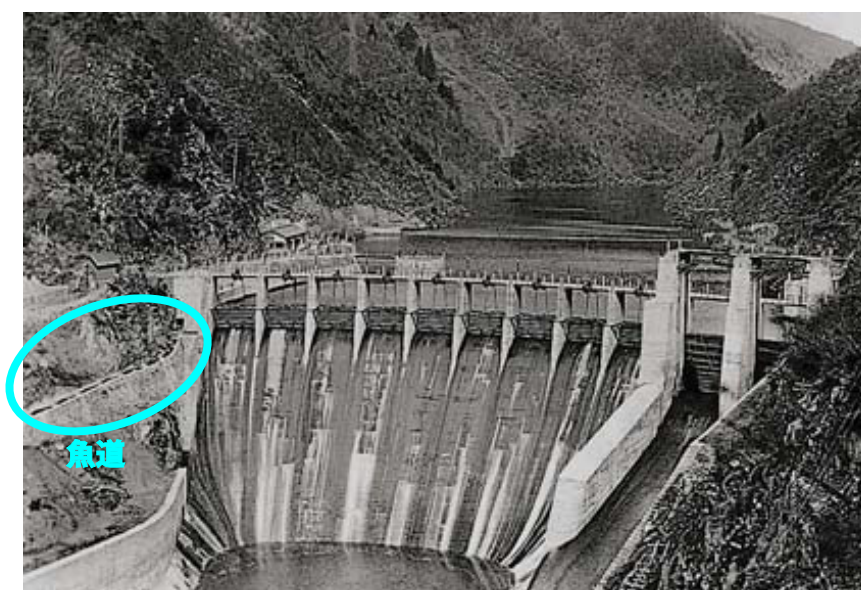
写真 1.3-5 大峯ダム概観 14)
