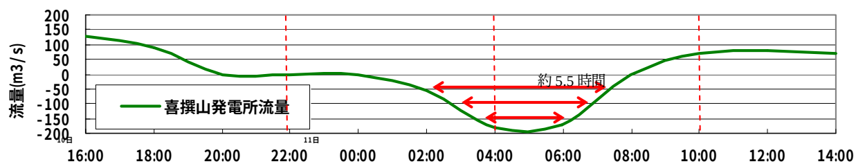
図 1.3-9 逆流の発生時間（天ヶ瀬ダム流入量が 35m³/s の場合）
