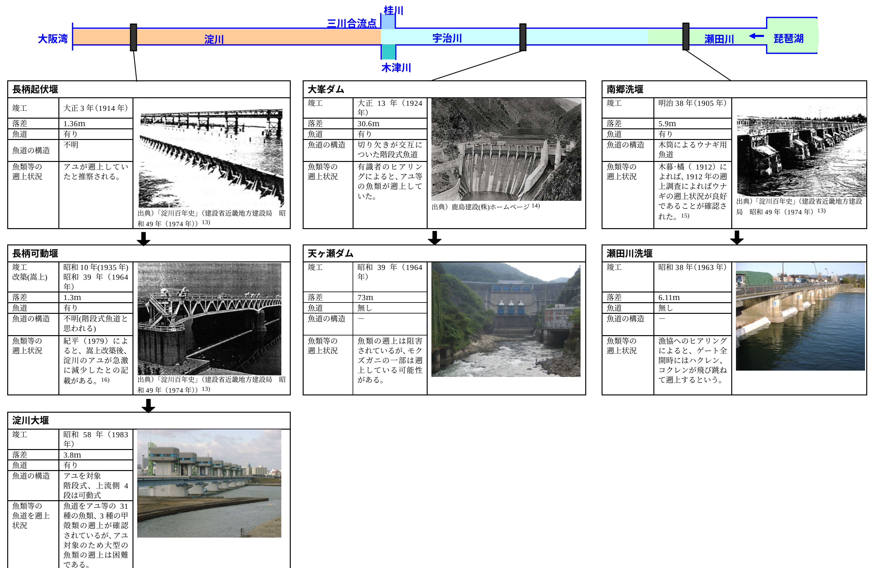
図 1.3-10 河川横断工作物の設置状況の変遷
